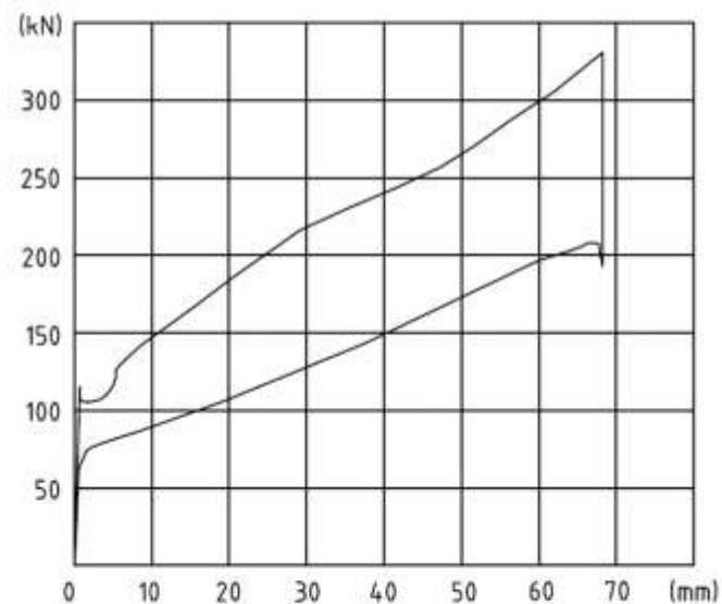
Charakterystyka statyczna
