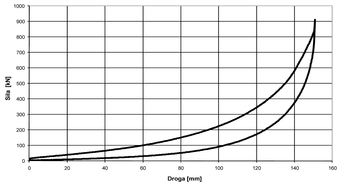
Charakterystyka statyczna
