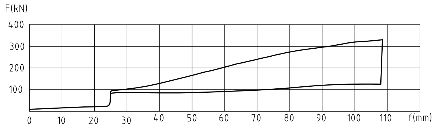
Charakterystyka statyczna
